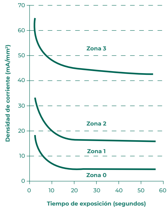
Figura 1. Efecto de la corriente sobre la piel dependiendo de la densidad de corriente y el tiempo de exposición
